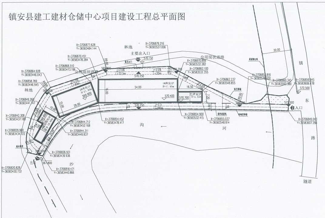
总平面图
